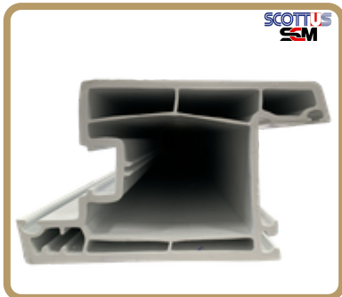
DAUN PINTU Z (Buka Dalam)
